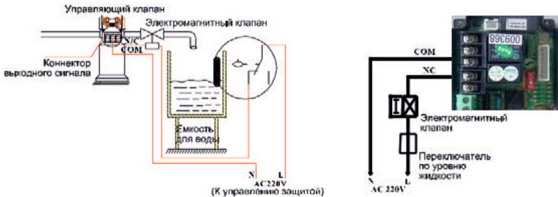
Рис. 3-1 Сеть управления электромагнитным клапаном на выходе
